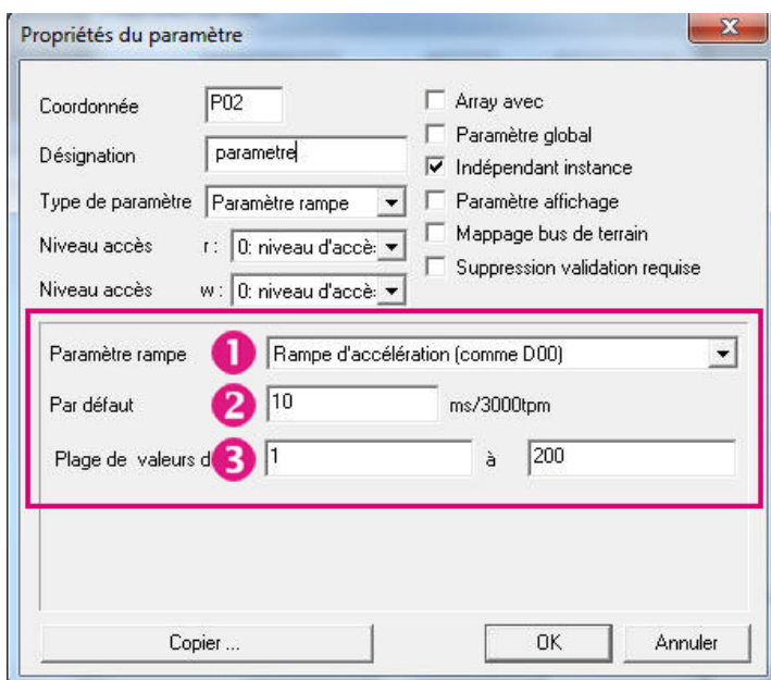
Fig. 4-7 Définition d'un paramètre rampe
