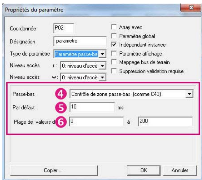
Fig. 4-8 Définition d'un paramètre passe-bas
