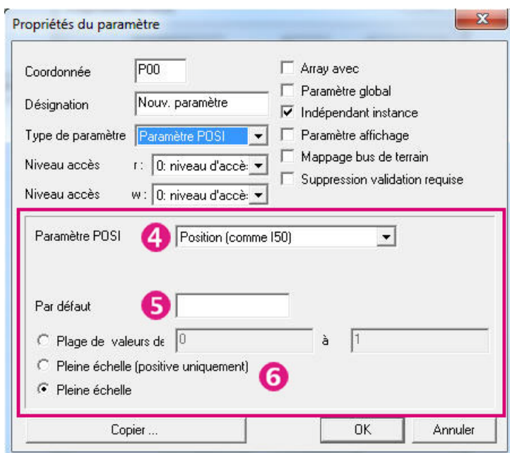
Fig. 4-11 Définition d'un paramètre POSI
